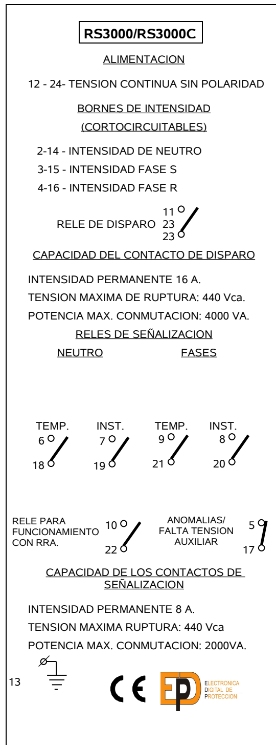
Fig.3 Etiqueta de embornamiento. Siempre situada en el lateral de la caja.
