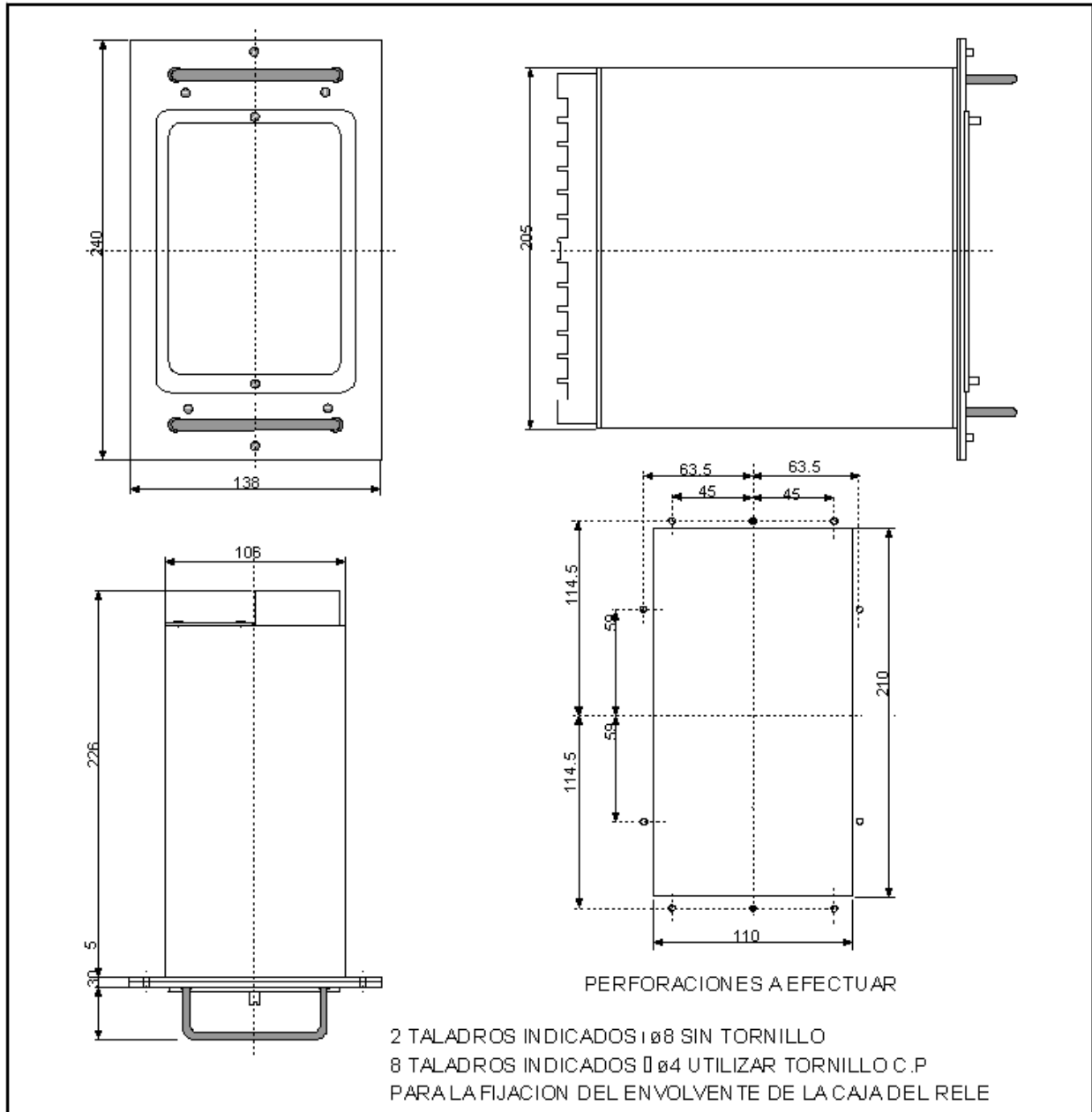
Fig.1 Dimensiones caja tipo B
